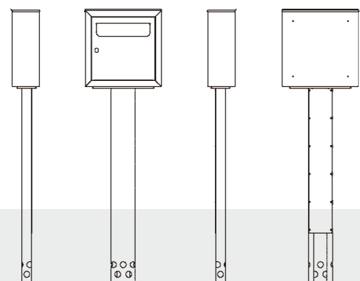
Mål POP 33 Udvendige mål: h x b x d = 470 mm x 470 mm x 170 mm Brevindkast: h x b = 33 mm x 325 mm
