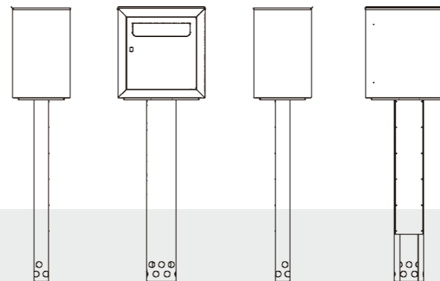
Mål POP 101 Udvendige mål: h x b x d = 555 mm x 545 mm x 360 mm Brevindkast: h x b = 36 mm x 360 mm
