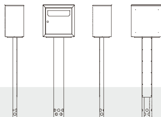
Mål POP 55 Udvendige mål: h x b x d = 470 mm x 470 mm x 280 mm Brevindkast: h x b = 36 mm x 325 mm
